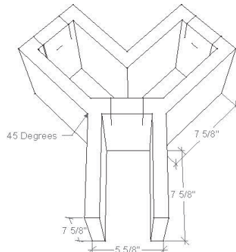
6x8x16 Y BLOCK
